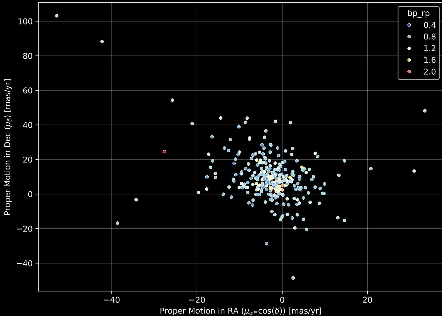
GALAH DR4 Field: [1552] Proper Motion Diagram (n= 286)
