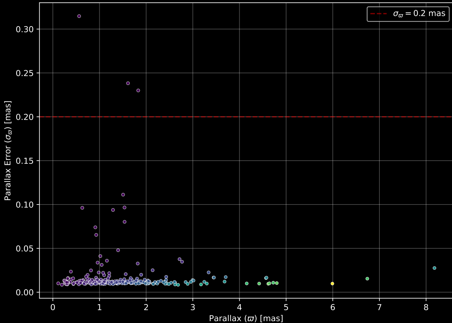
GALAH DR4 Field: [1552] Parallax Quality (n= 286)
