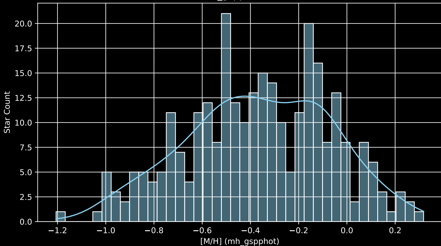
GALAH DR4 Field: [1552] [M/H] (mh_gspphot) (n= 286)
