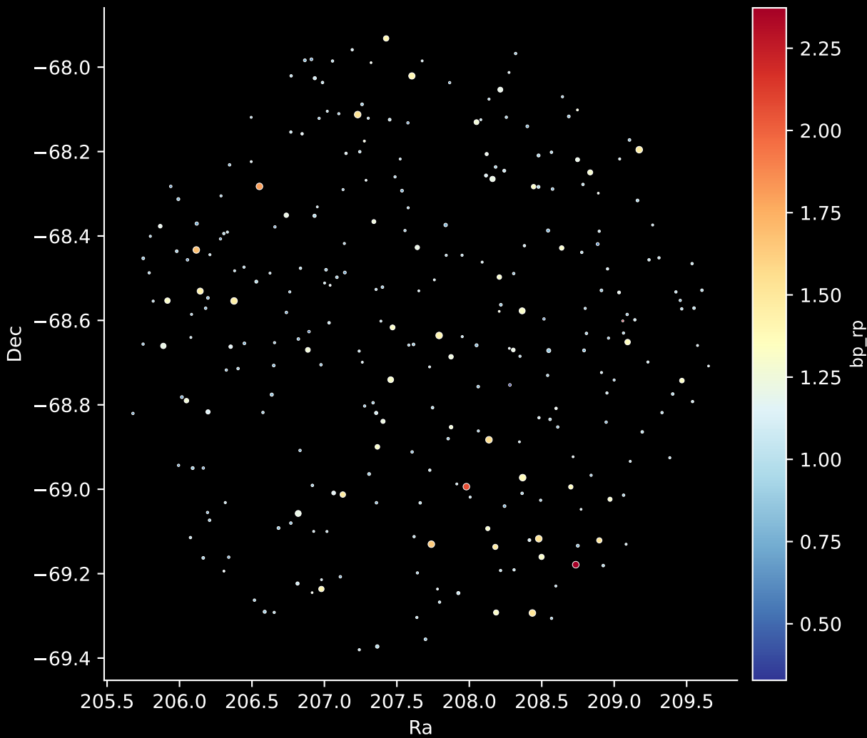
GALAH DR4 Field: [1552] Stars: 286
